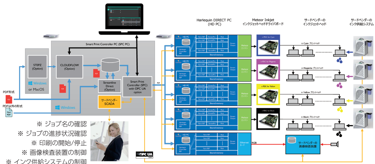
ケース1: SmartDFE (CMYK、片面印刷、画像検査装置付)フルバリエーション対応の例
